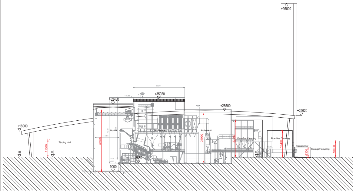
Section A-A 1:500
