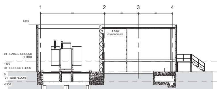
Section B 1 : 100
