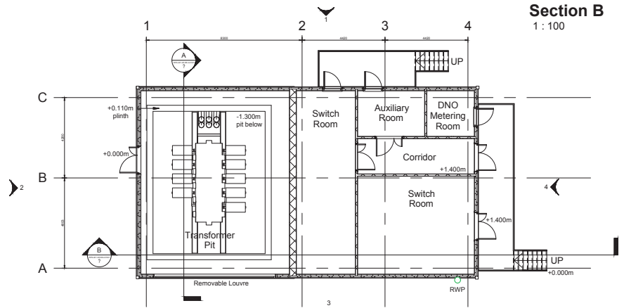
HV/LV Layout Plan 1 : 100
