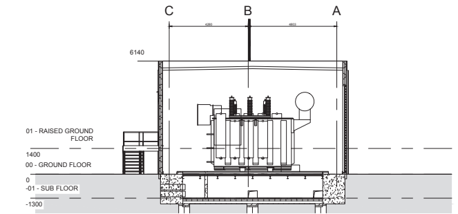
Section A 1 : 100
