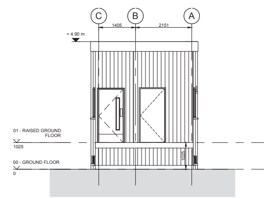
Section A-A 1 : 50
